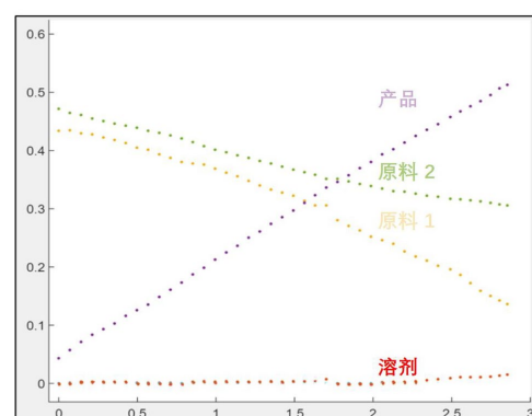
反应趋势
